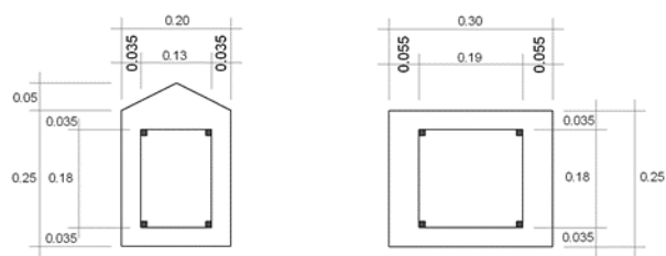
SECCION A-A SIN ESCALA SECCION B-B ESCALA 1:100 DETALLE DE POZO REFORZADO PARA AGUAS LLUVIAS
