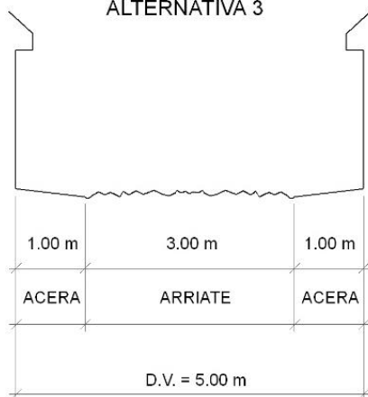
ALTERNATIVA 3
