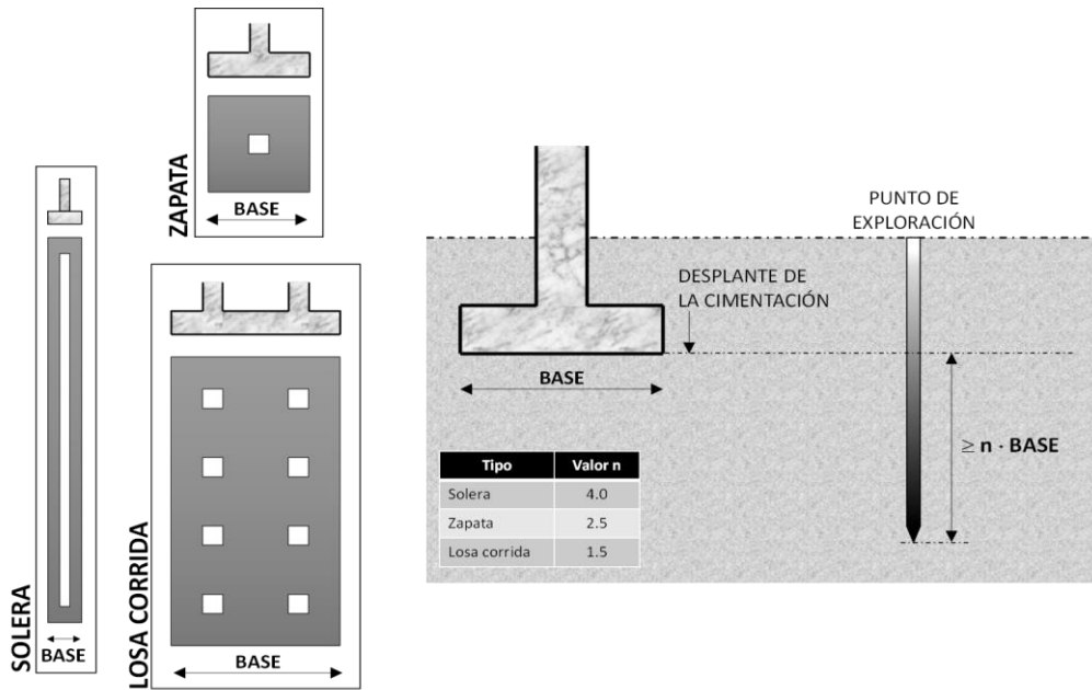
Figura 4.4 Profundidad respecto a cimentaciones superficiales
