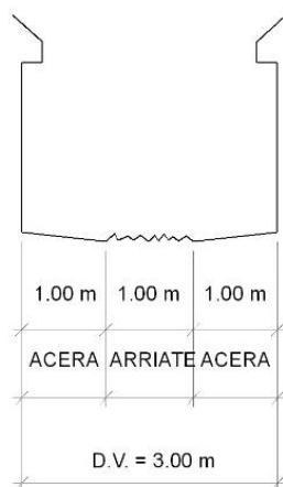
ALTERNATIVA 1
